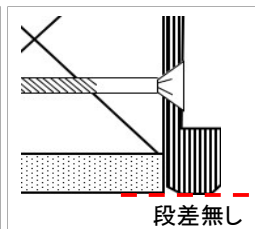
縦柵下地の見込寸法は壁厚同等
