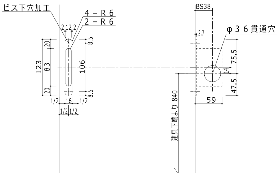
【錠加工】※床仕上げ面より鍵錠センター 850 mm の場合 ※アウトセット片引き戸【エンド枠なしタイプ】 は戸先に錠は付きません。
