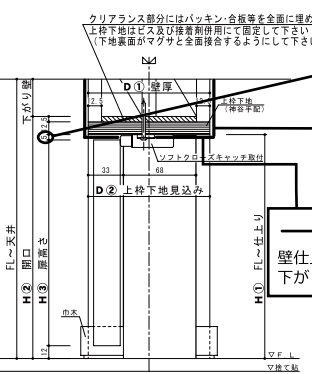
下がり壁納まり
