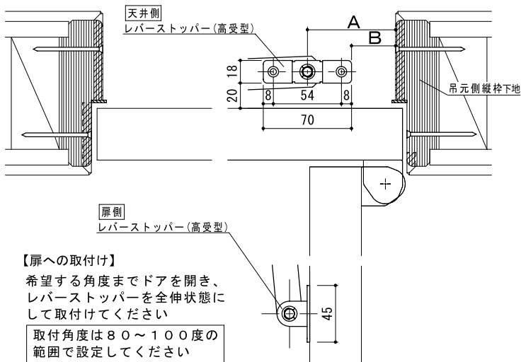
縦断面図
