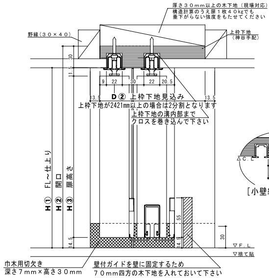
天井高納まり
