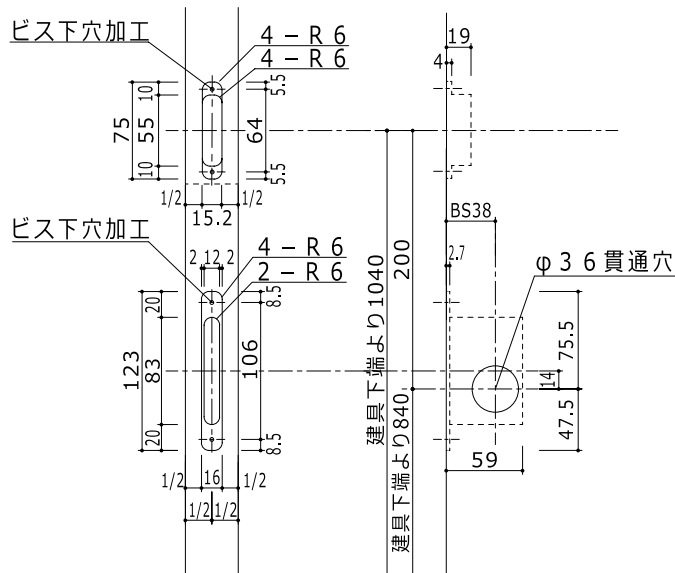
【錠付き】※床仕上げ面より鍵錠センター 850 mm の場合
