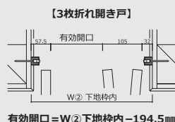
〔3枚折れ開き戸有効開口〕
