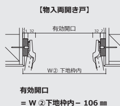
〔物入開き戸有効開口〕
