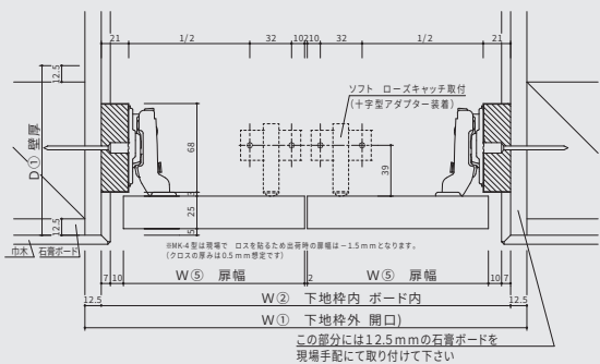
〔横断面〕
