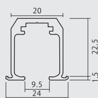
[引込みポケット戸 (上吊)]
