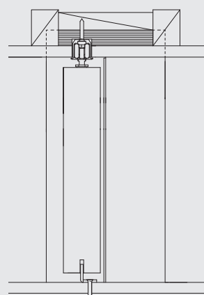
[納まり図・ 実寸平面図] QR
