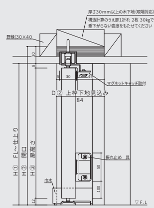
〔縦断面〕
