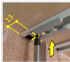
上部ストッパーを 上レールに取付ける
