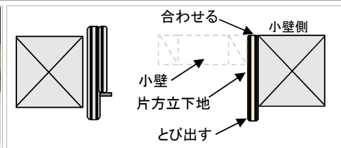
片方立下地の取り付け位置 (小壁側の壁面と下地材を合わせる)
