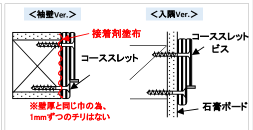
【準耐火納まりの場合】 コーススレットビスで固定(2mmクリアランスは無)入隅の場合、石膏ボードの上に縦枠を取付け
