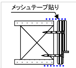
メッシュテープ貼り (石膏ボードと枠をまたぐように貼る)
