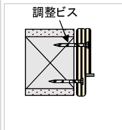
調整ビスにより枠を固定
