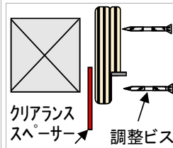
クリアランス スペーサーを挟む
