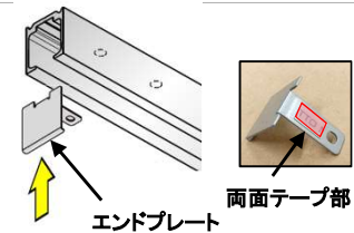
エンドプレートを両面テープで仮止めし、 上レールと一緒に固定する
