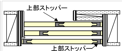
上部ストッパーの取り付け位置
