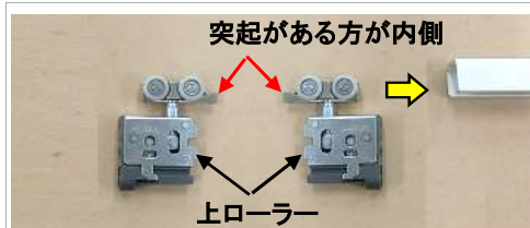
上ローラーを上レールに入れる
