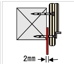
2mmのクリアランスを保ち調整ビスにより枠固定
