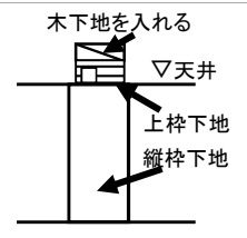
上枠下地の裏には木下地を入れる
