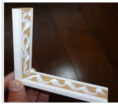
接着剤全面塗布
