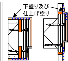
パテ処理
