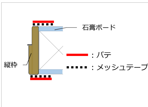
ジョイント部をまたいでメッシュテープを貼る
