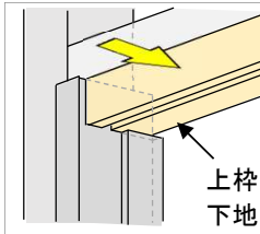
上枠を縦枠勝ちに納める
