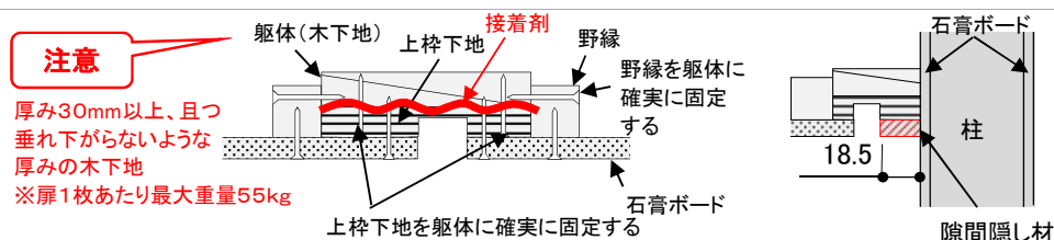
上枠下地取付け位置 (中方立下地から41mm)
