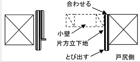
片方立下地の取付け位置
