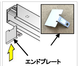
上レール両端にエンドプレートを両面テープで仮止めし、上レールと一緒に固定する
