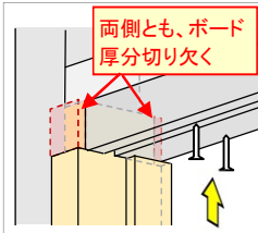
下地表よりビス固定
