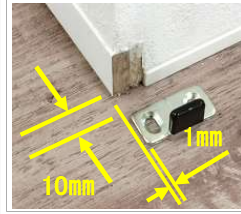
床付ガイドの取付け
