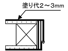
塗り代2～3mm
