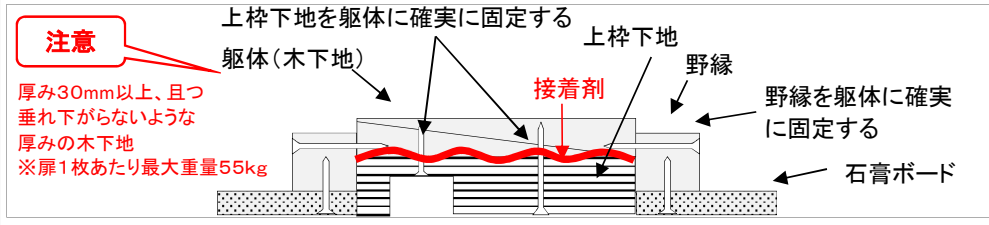
石膏ボードの厚さ分を確保して、野縁を躯体に固定 その後、野縁に石膏ボードを取付ける
