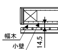
下部レール(ガイドは使用不可)
