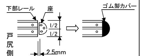
下部戸当たりの取付
