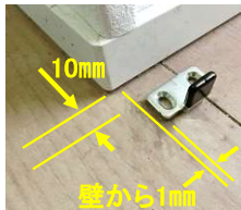
床付ガイドの場合
