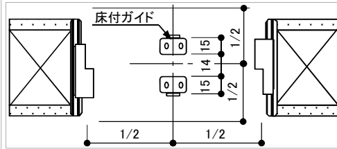
床付ガイドの取り付け
