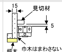
【準耐火(15mmボード)の場合】 壁付用下部固定金具の取付け ※幅木は廻さずかい木も使用しない
