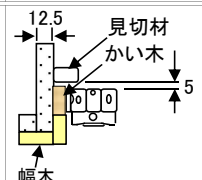
【標準(12.5mmボード)の場合】 厚み5.5～7mm×巾22mm×高さ61mmのかい木を当て壁付用下部固定金具を取付
