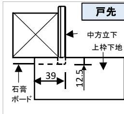
上枠下地取付位置 (中方立下地から39mm)
