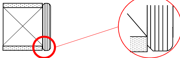
中方立下地は面取りされている側を石膏ボードと接合させる
