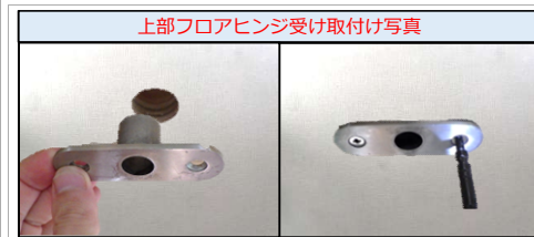
穴加工部に上部フロアヒンジ受けを 同梱ビス（M5×25 半ネジ）で取付け
