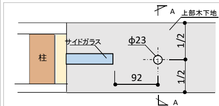
【吊元側サイドガラスの場合】 サイドガラス端部から92mmの位置に穴加工
