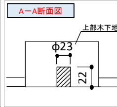
穴加工断面寸法 φ23 深さ22mm
