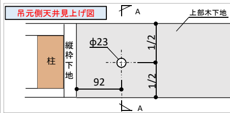
穴加工位置
