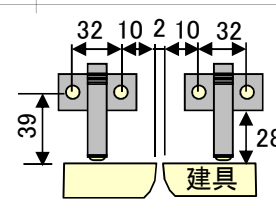
取り付け位置（両開き）
