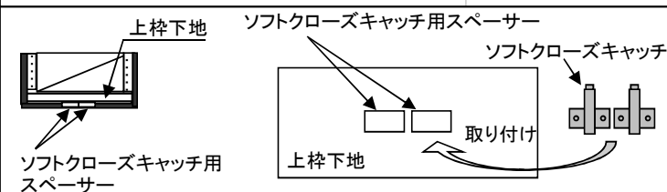
ソフトクローズキャッチをソフトクローズキャッチ用スペーサーの上から取り付け
