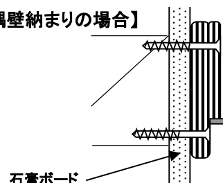
コーススレッドビスで建枠下地を取付
