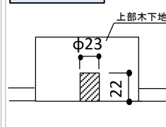
穴加工断面寸法 φ23 深さ22mm
