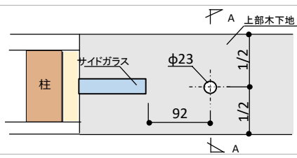
穴加工位置
