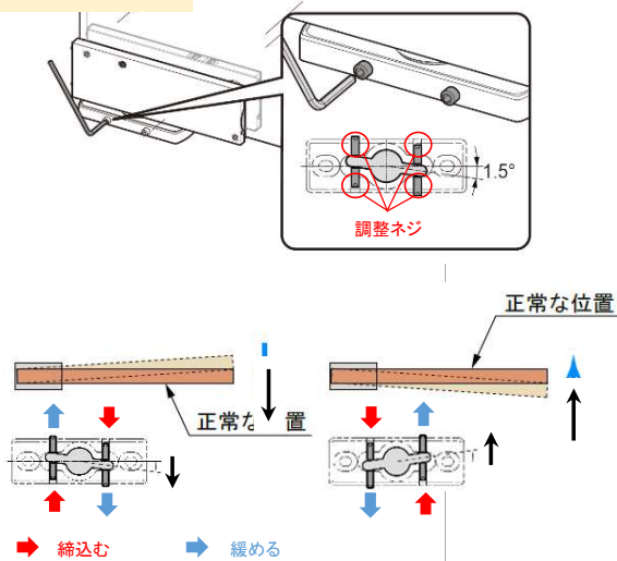
扉の閉鎖位置調整
