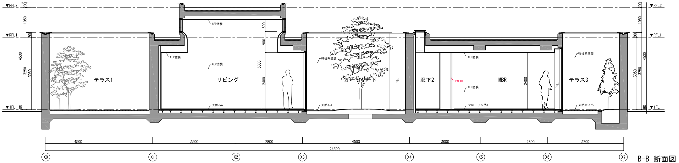
B-B 断面図
