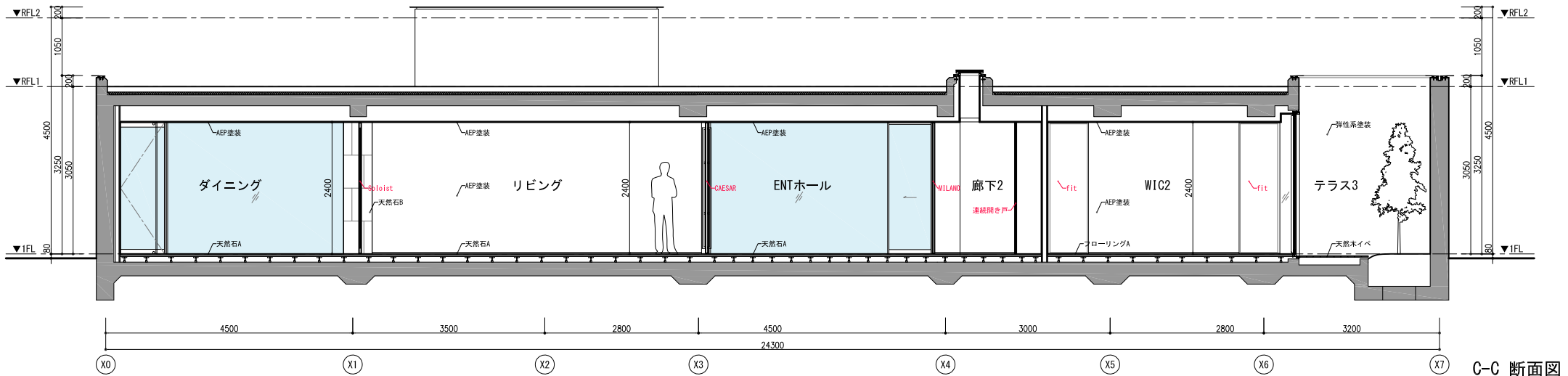
C-C 断面図
