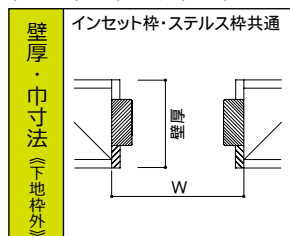
物入両開き戸・片開き戸
