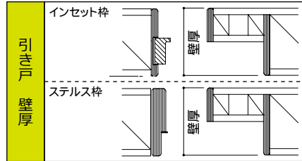
片引き戸・2枚(3枚)引込み戸
