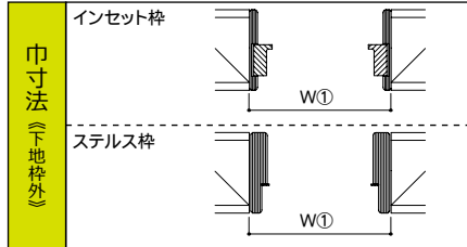
片開き戸・親子戸・2枚(3枚)引違戸
